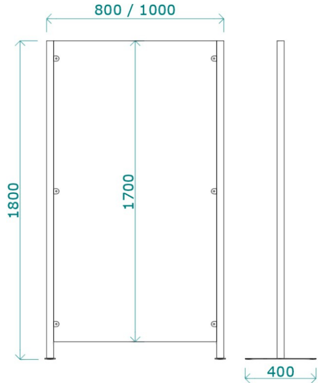
Dimensiones
